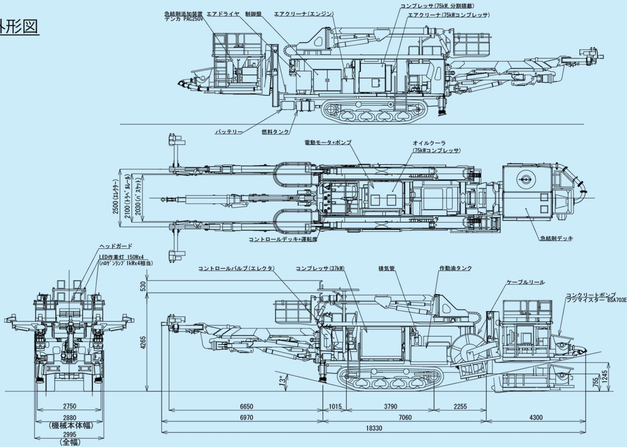
エレクター・バスケット正面図
