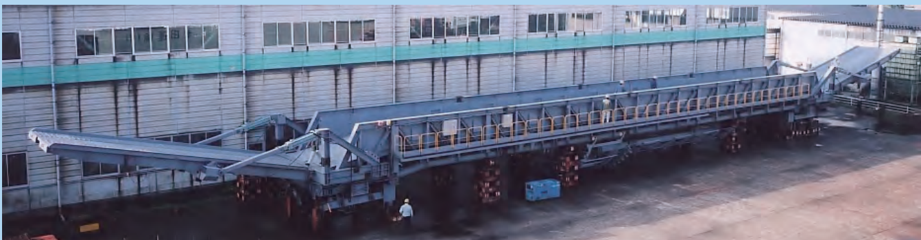
移動棧橋（標準 3 スパンタイプ）
